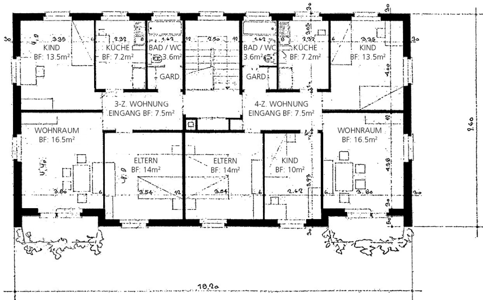
Grundrissplan OG - Haus 10 / 12 / 14 - nicht masstabsgetreu
